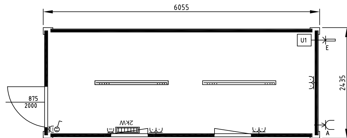
RCB20 - Büromodul - Rechtsseitig
