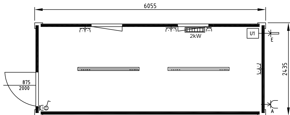
RCB20 - Büromodul - Linksseitig
