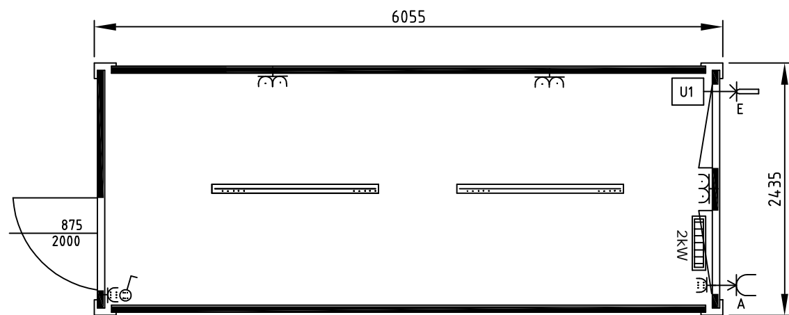
RCB20 - Büromodul - Stirnseitig
