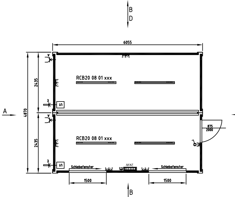
Ansicht A
